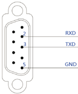
COM1/2/3/4/5/6-RS232 接口定义
